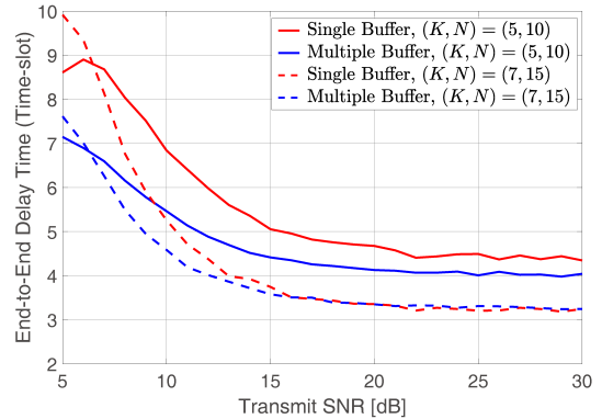
그림 1 중계 협력 시스템에서 다중 버퍼와 단일 버퍼의 종단 지연 성능
