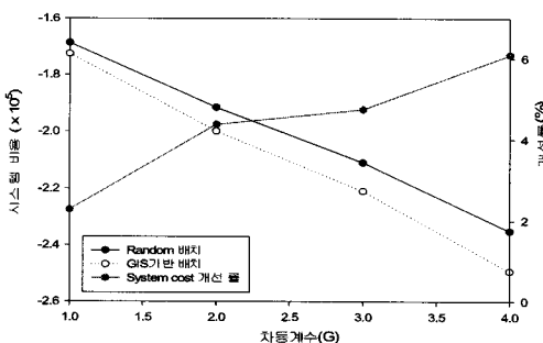
그림 8. G변화에 따른 초기 시스템 비용(n=1)
