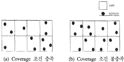
그림 2. 센서 배치에 따른 Coverage 조건의 가부
