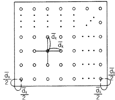
그림 4. 전체영역에서의 센서 초기 배치도 예
