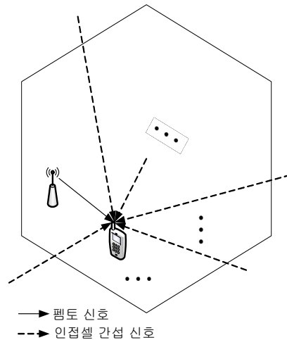
그림 1. 시스템 모델 Fig. 1 System Model
